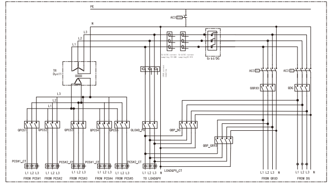
STS250D CABINET
